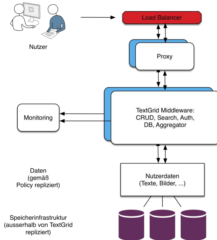
Abbildung 2: Grundkonzept der Hochverfügbarkeit
